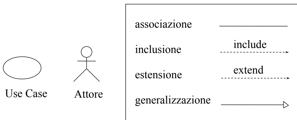
Relazioni nel diagramma degli use case
