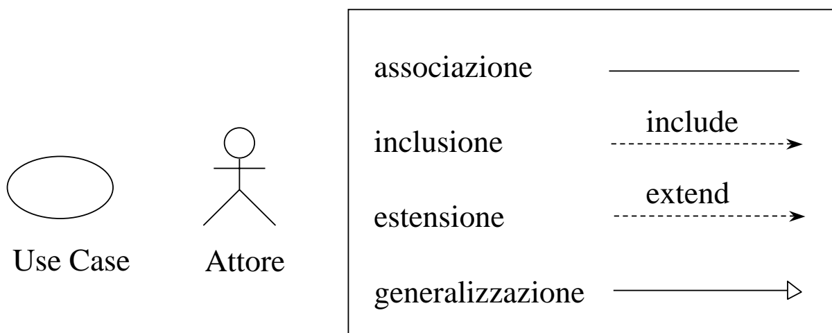
Relazioni nel diagramma degli use case
