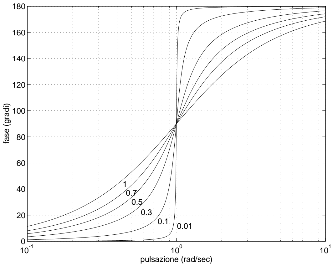
Termine trinomio a numeratore ( \omega_n = 1 ): diagrammi di Bode al variare dello smorzamento \zeta .
